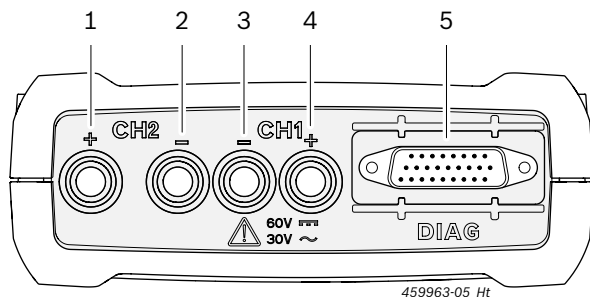
Abb. 2: Diagnostikariba/mõõteriba KTS 590
