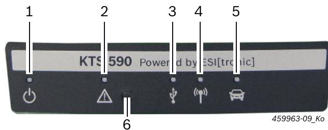
Abb. 5: LED állapotjelzés
