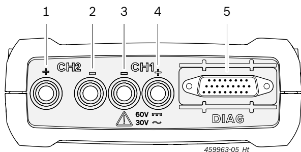
Abb. 2: Diagnostiikanastat/mittaustulot KTS 590
