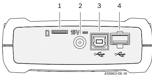
Abb. 3: Jungčių blokas
