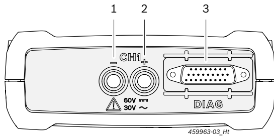
Abb. 1: Diagnostična letev/merilna letev KTS 560
