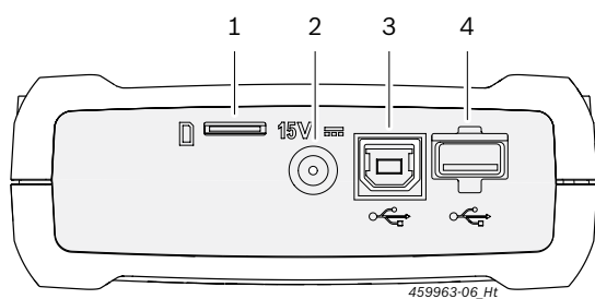
Abb. 3: Ühendusriba
