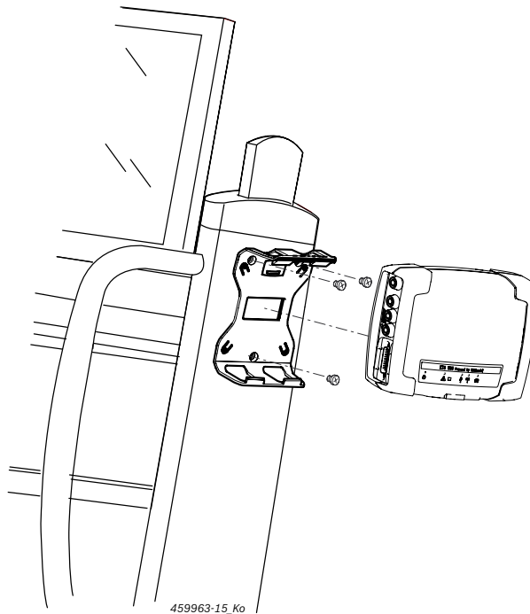
Abb. 7: Montage Befestigungshalter
