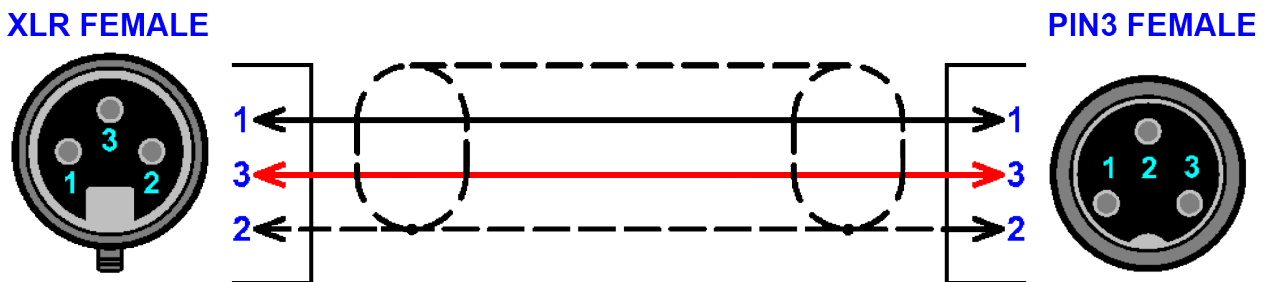
Универсальный кабель для USB Autoscope IV.
