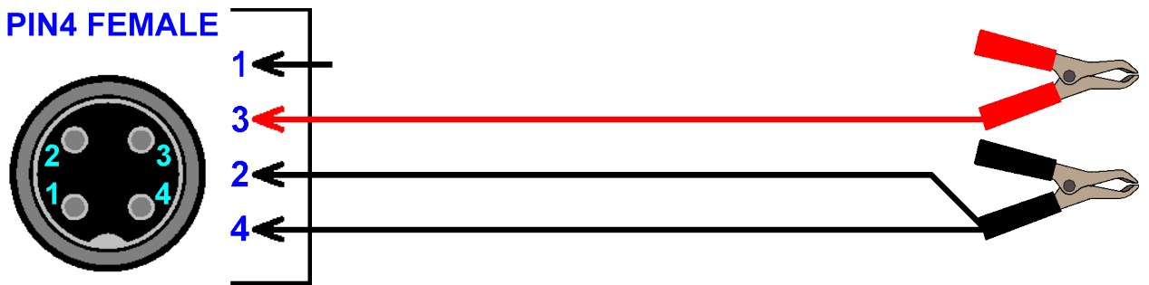
Питающий кабель USB Autoscope IV.
